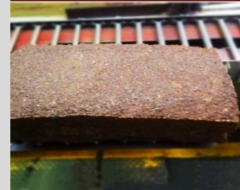
Crumb Rubber
